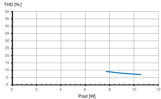
Factor total armónico / Total harmonic factor / Facteur harmonique total (THD)
