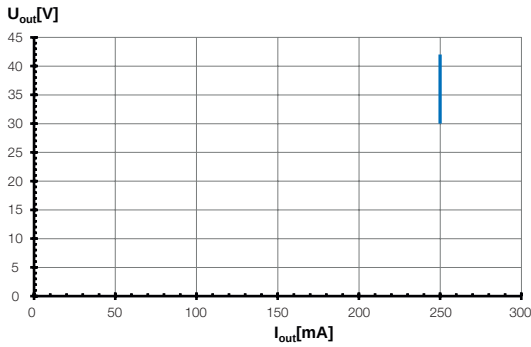
Área de trabajo / Working area / Zone de travail
